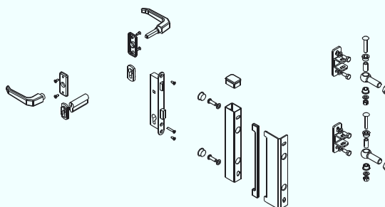
Rys. 6. Akcesoria furtki ręcznej().
