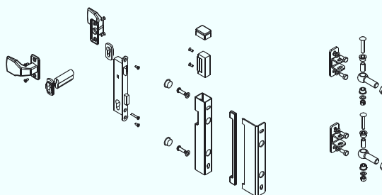
Rys. 7. Akcesoria furtki z elektrozaczepem.
